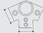
Stolpefot deksel
